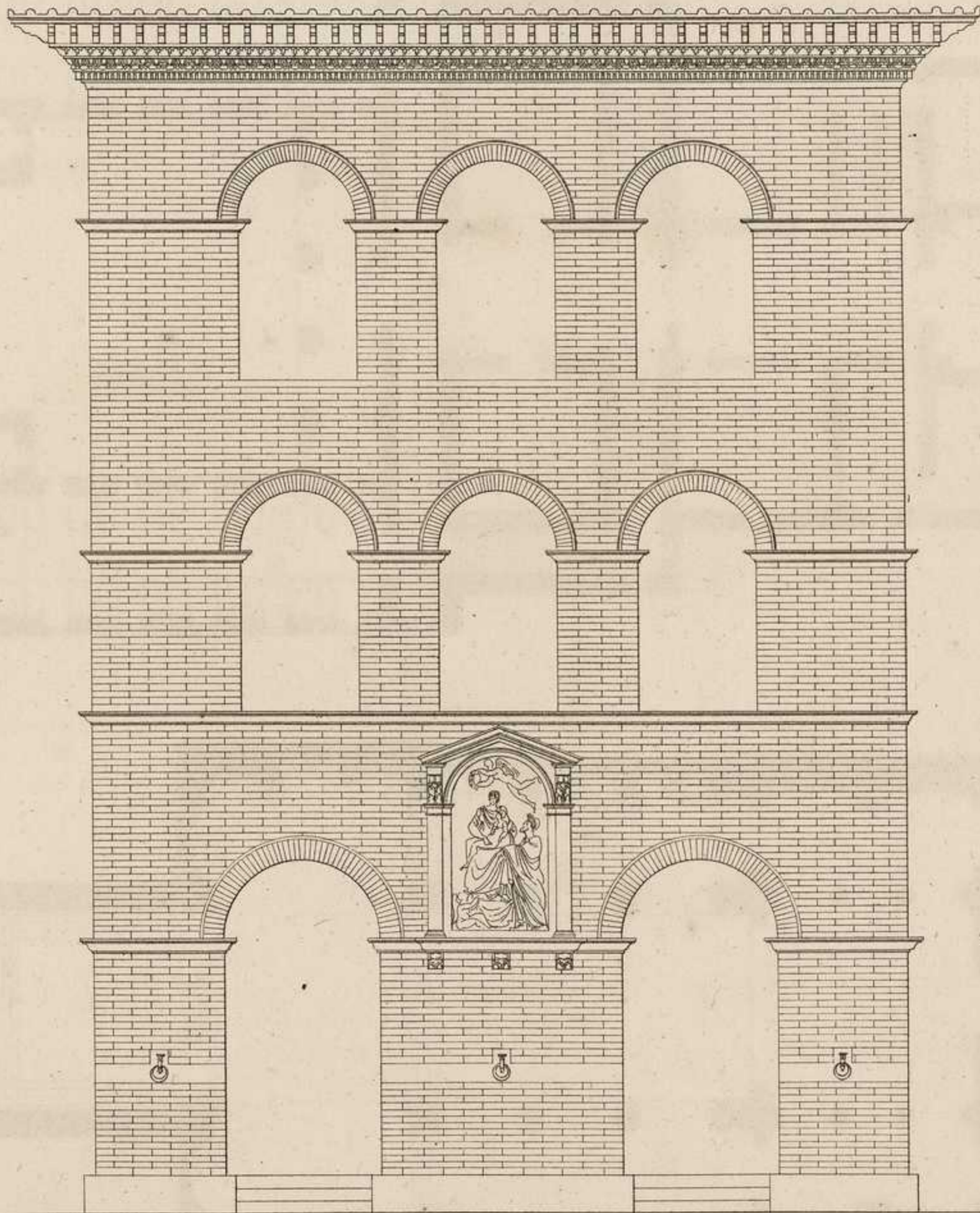
FACADE D'UNE MAISON, RUE DEL CORSO, A SIENNE.
