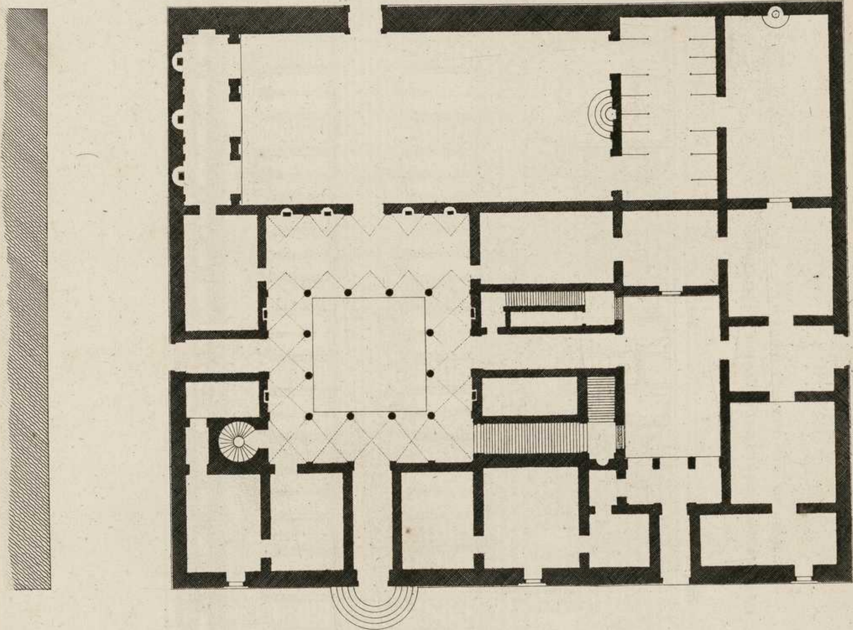
PLAN DU PALAIS RICARDI, AUTREFOIS MEDICIS DANS LA VIA LARGA
