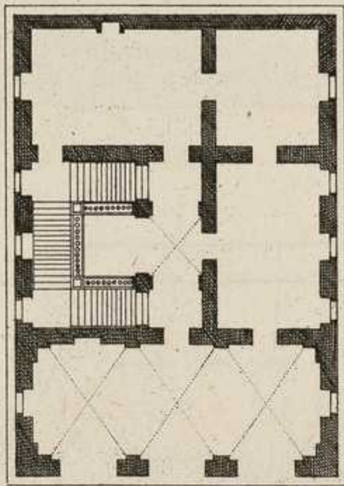
PLAN DU PALAIS COCCHI.
