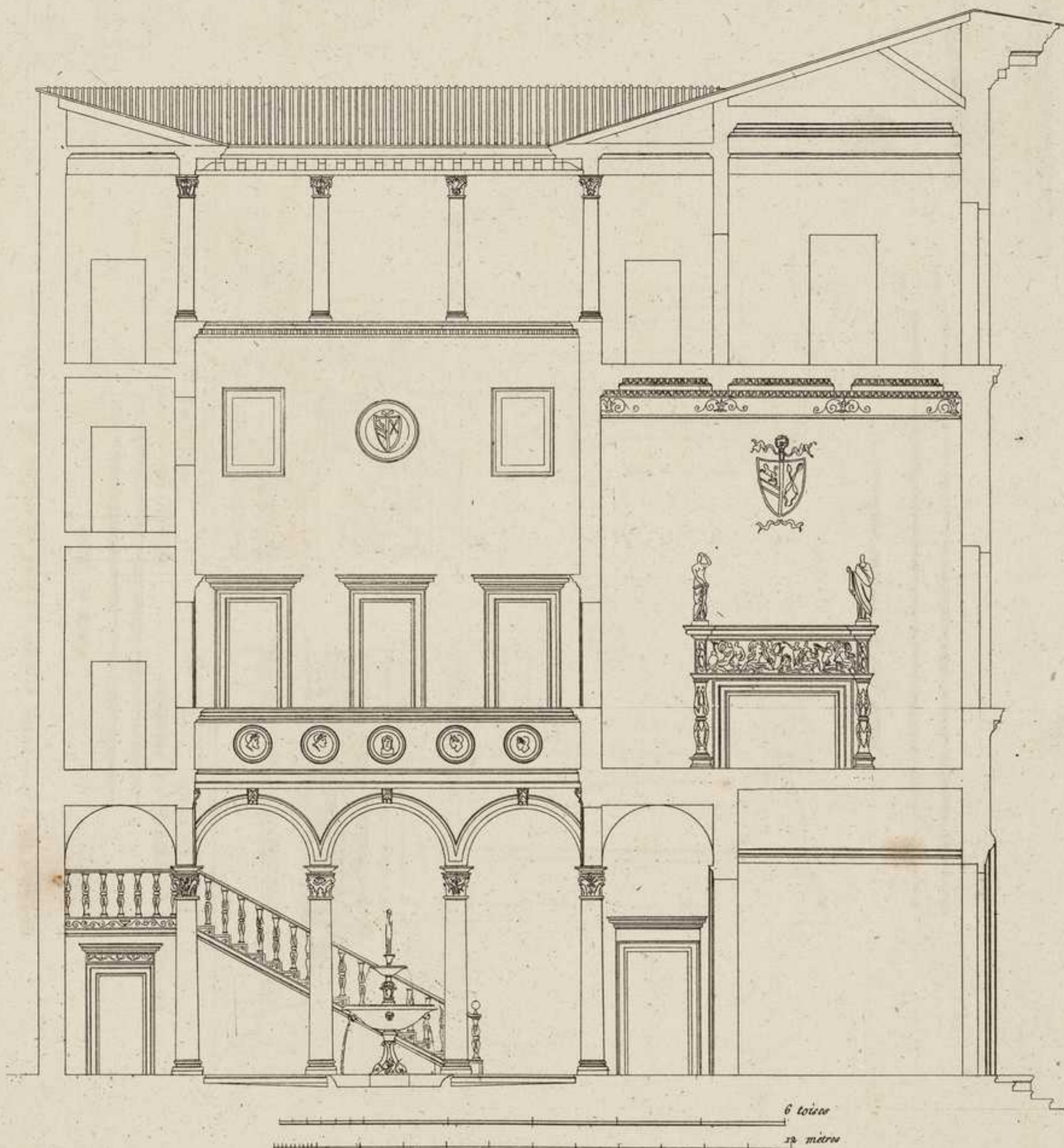
COUPE DU PALAIS GONDI, A FLORENCE.
