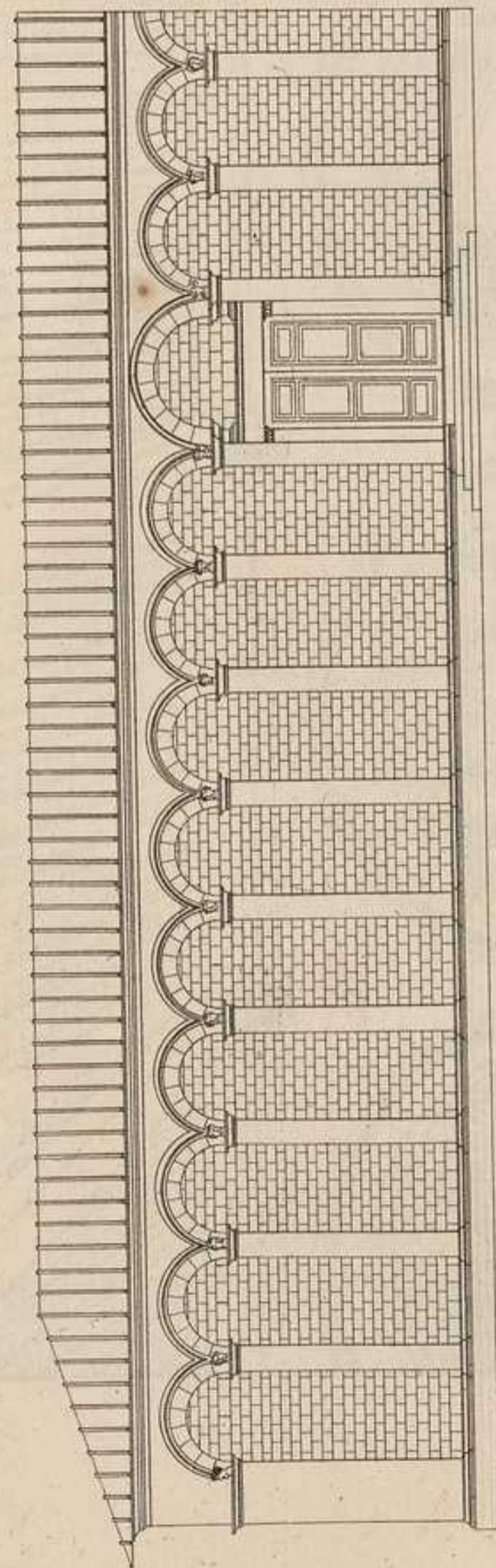
Détail du mur extérieur.
