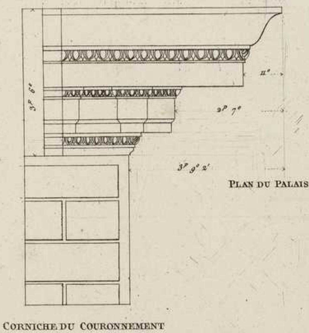
CORNICHE DU COURONNEMENT
