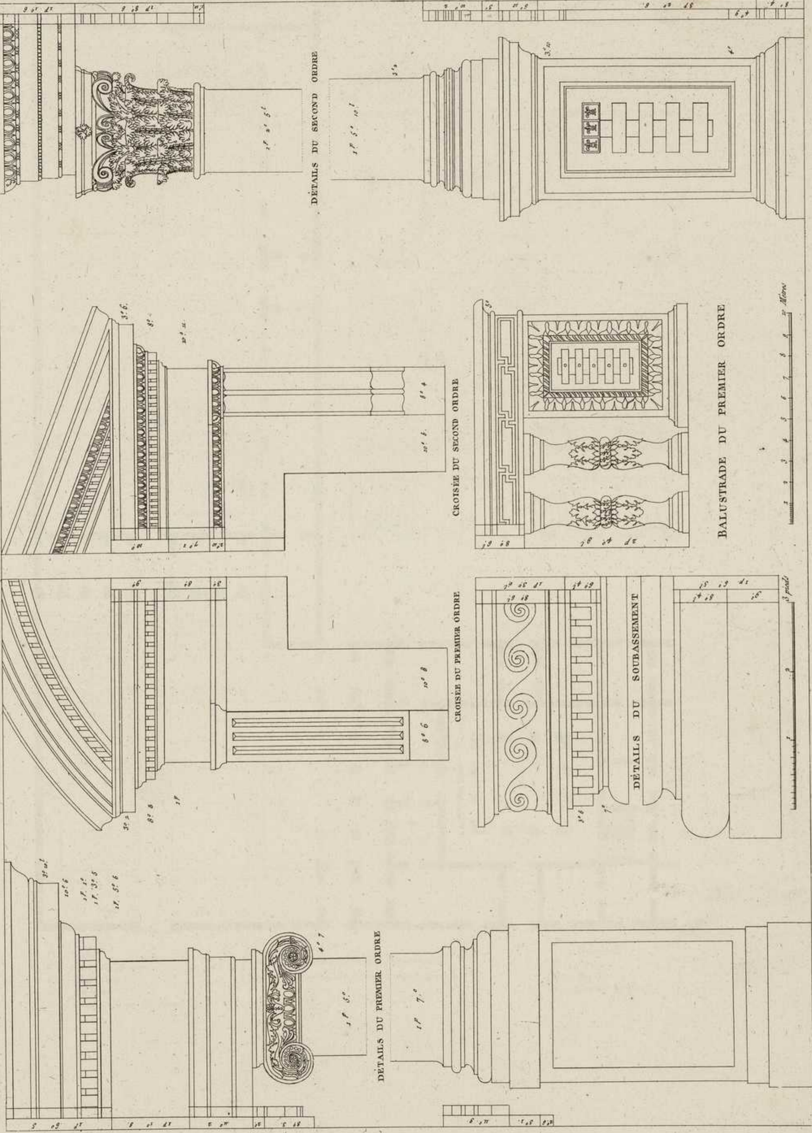
DÉTAILS DU PALAIS UGUCCIONI.
