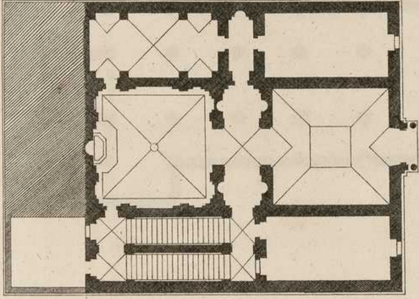
PLAN D'UN PETIT PALAIS A FLORENCE .
