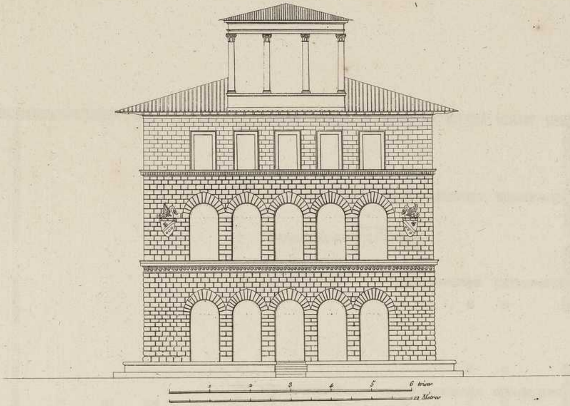
FAÇADE D'UN PALAIS VIA DEI PANDOLFINI, A FLORENCE
