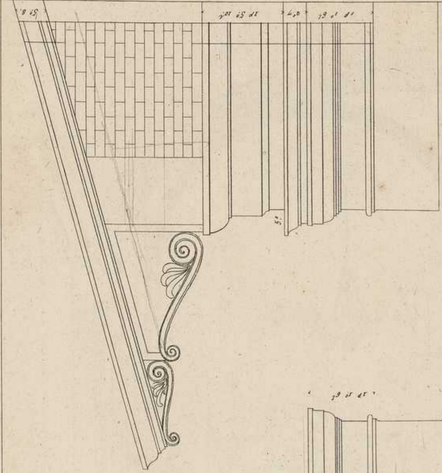
CORNICHE DU COURONNEMENT
