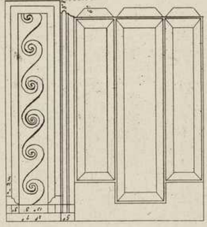
CORNICHE DU SOUBASSEMENT
