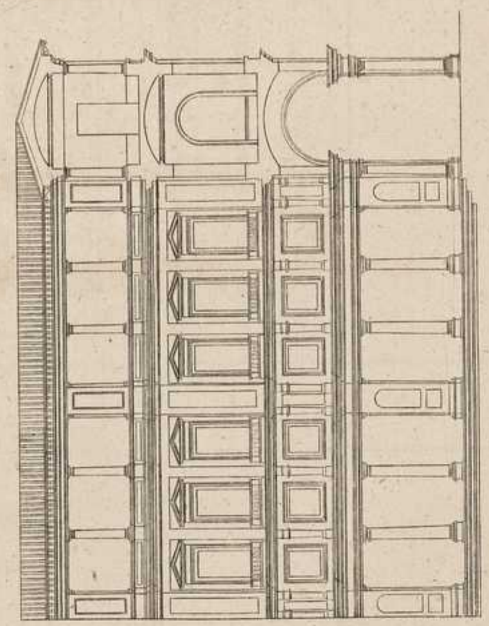
PORTION DE LA COUPE TRANSVERSALE DU PALAIS DES OFFICES.
