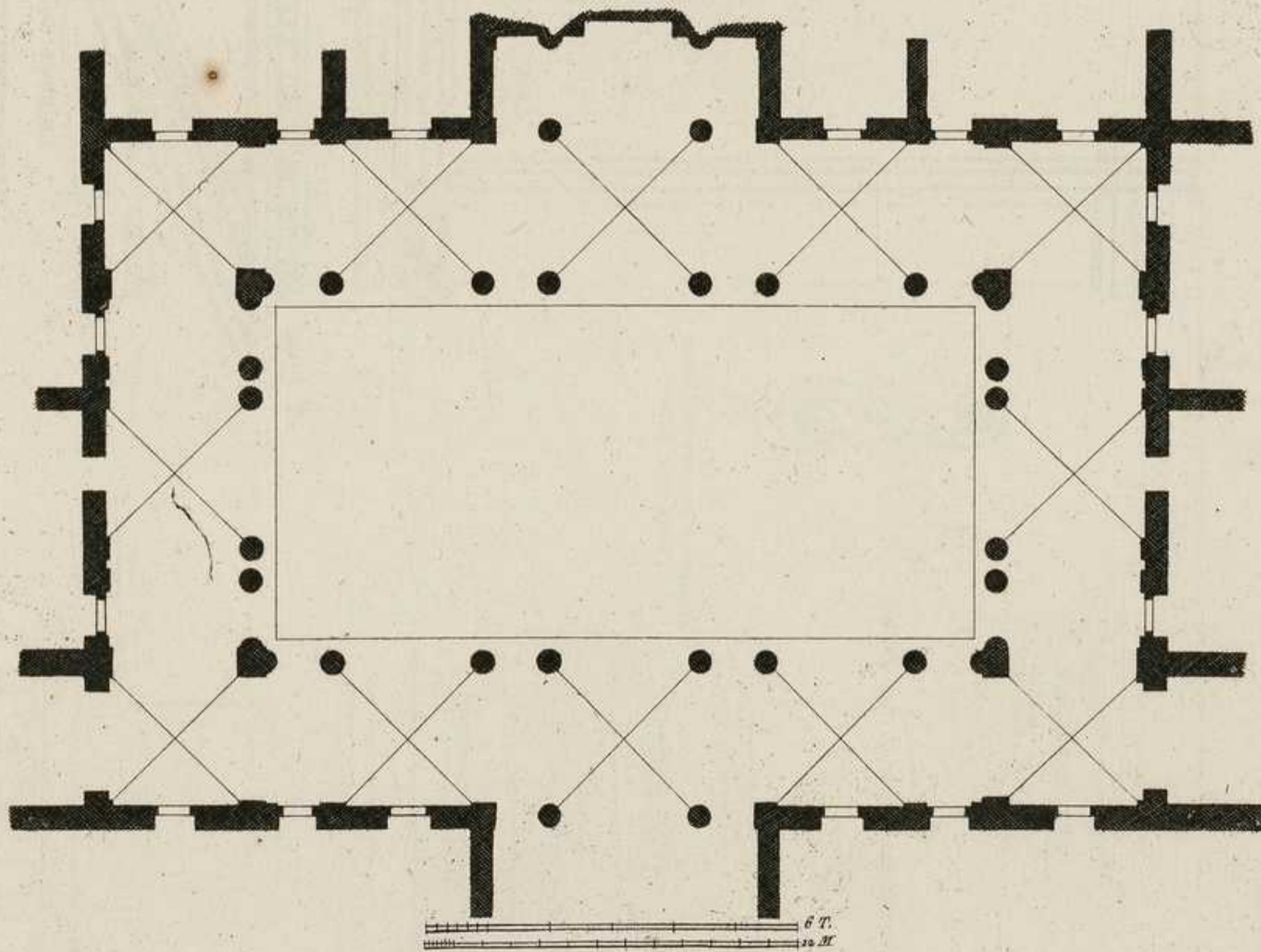
PLAN DE LA COUR DU PALAIS STROZZI.
