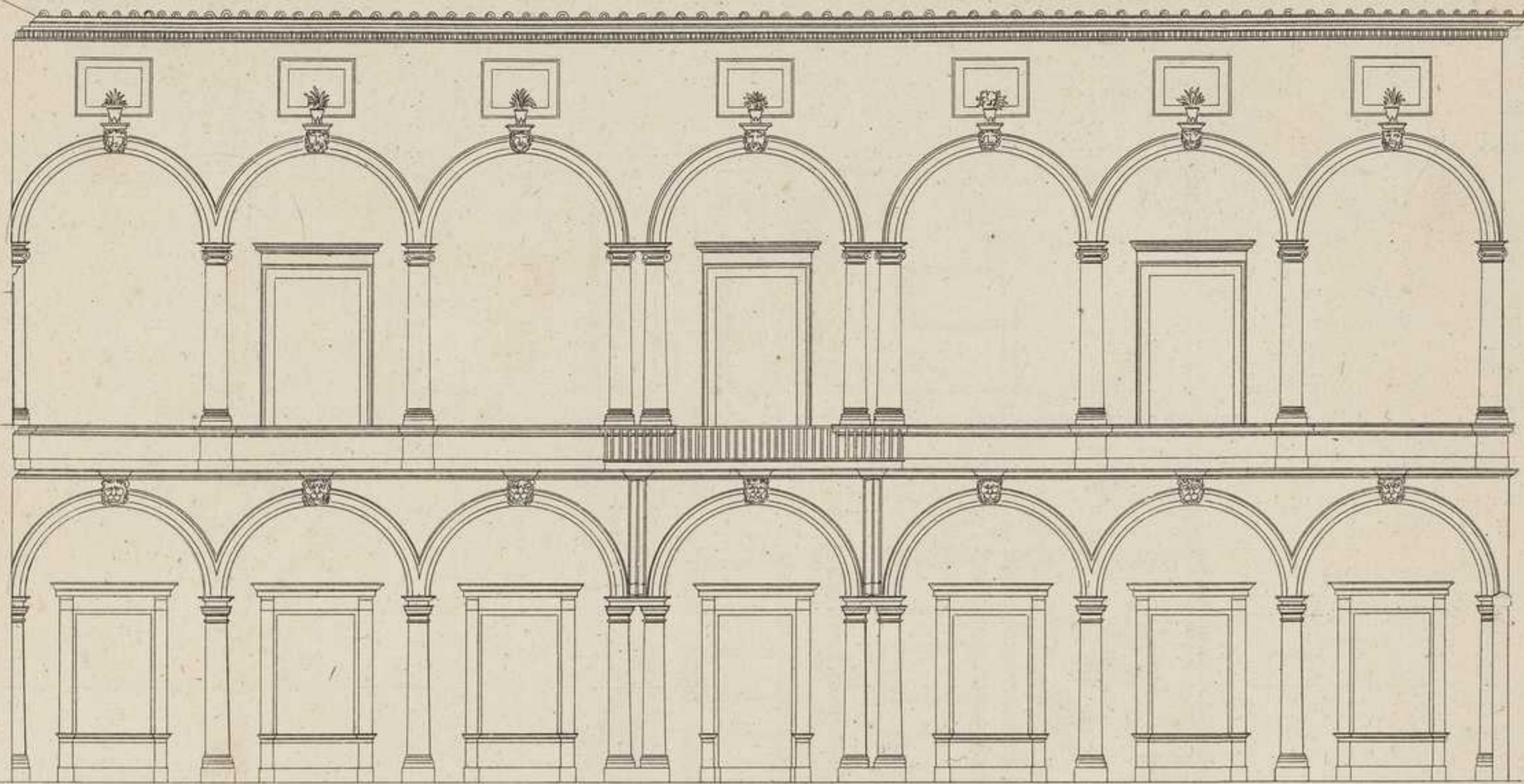
ELEVATION GEOMETRALE DU PALAIS NICOLINI, A FLORENCE
