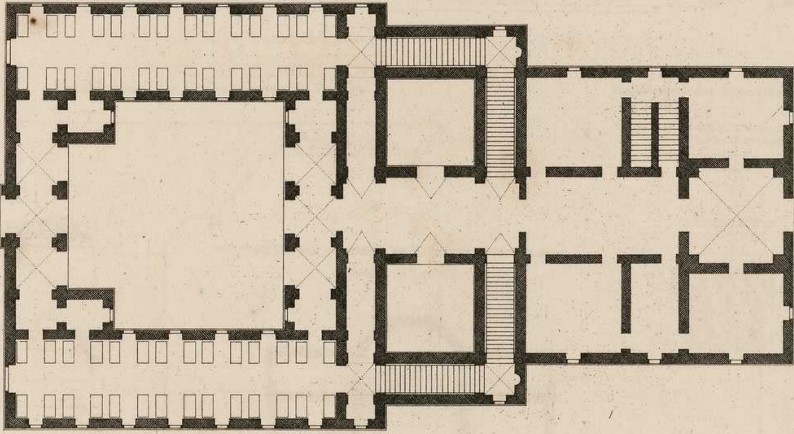
PLAN D'UN HÔPITAL, A AREZZO.
