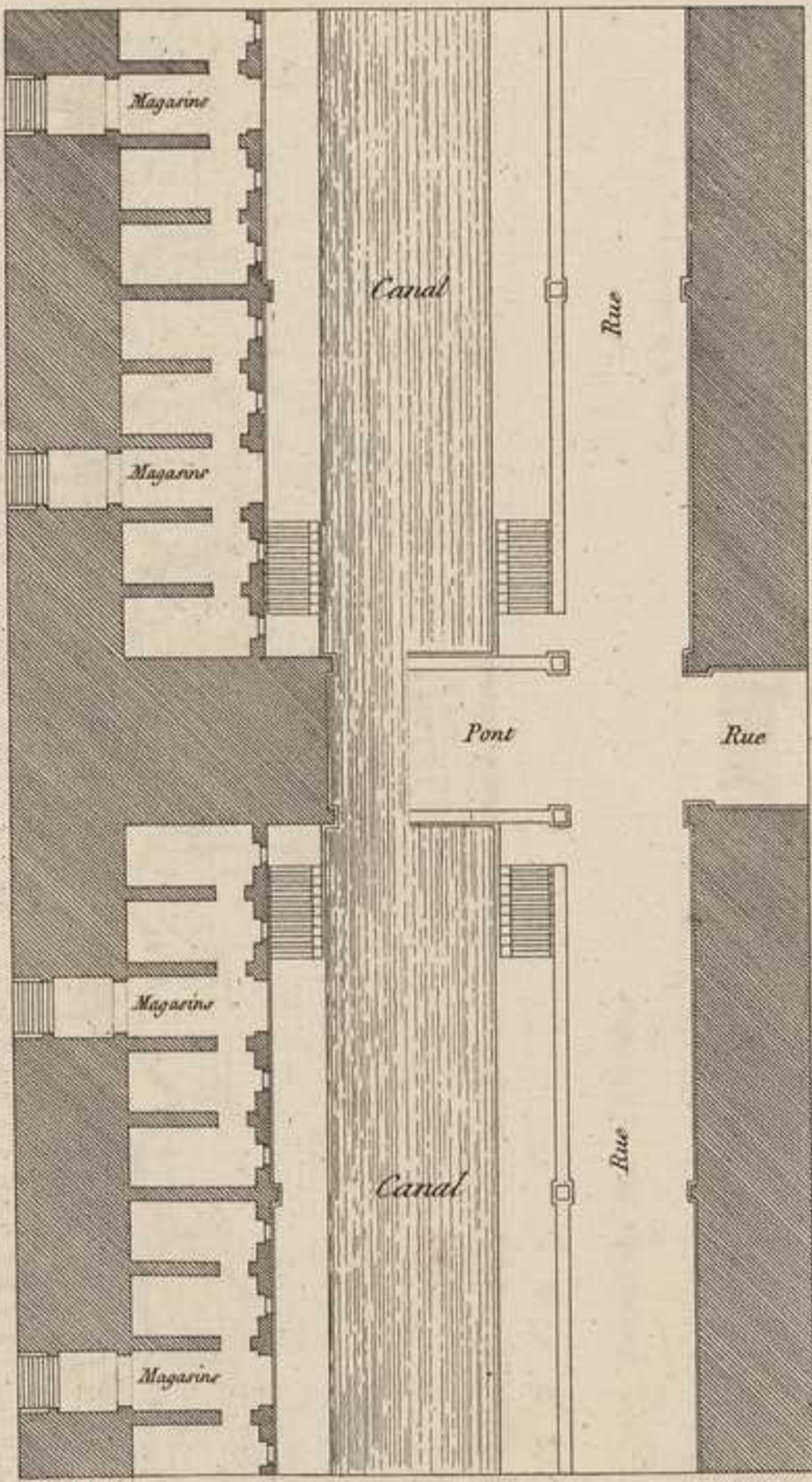
PLAN DE LA NOUVELLE VENISE.
