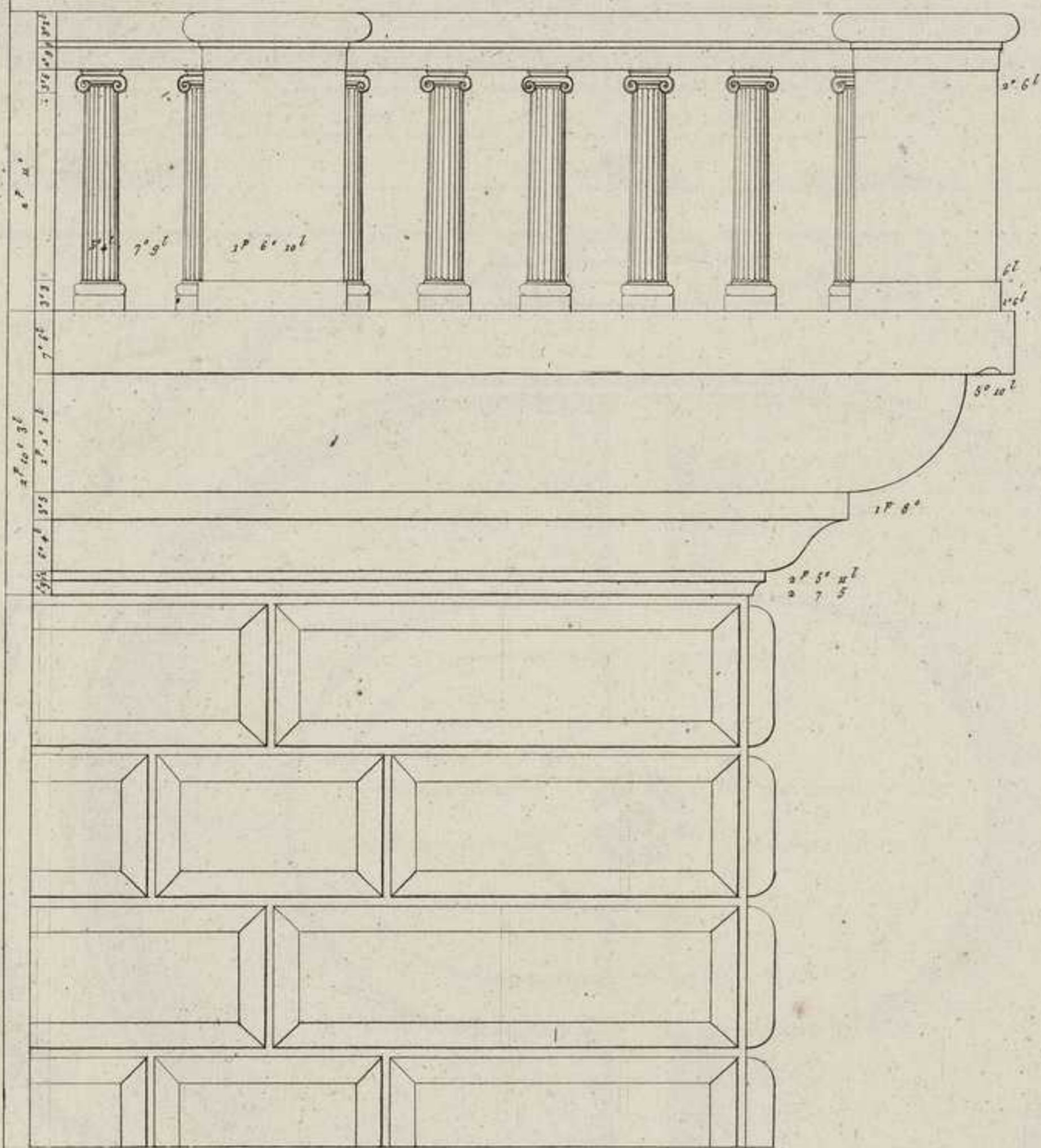
CORNICHE DU PALAIS PITTI.
