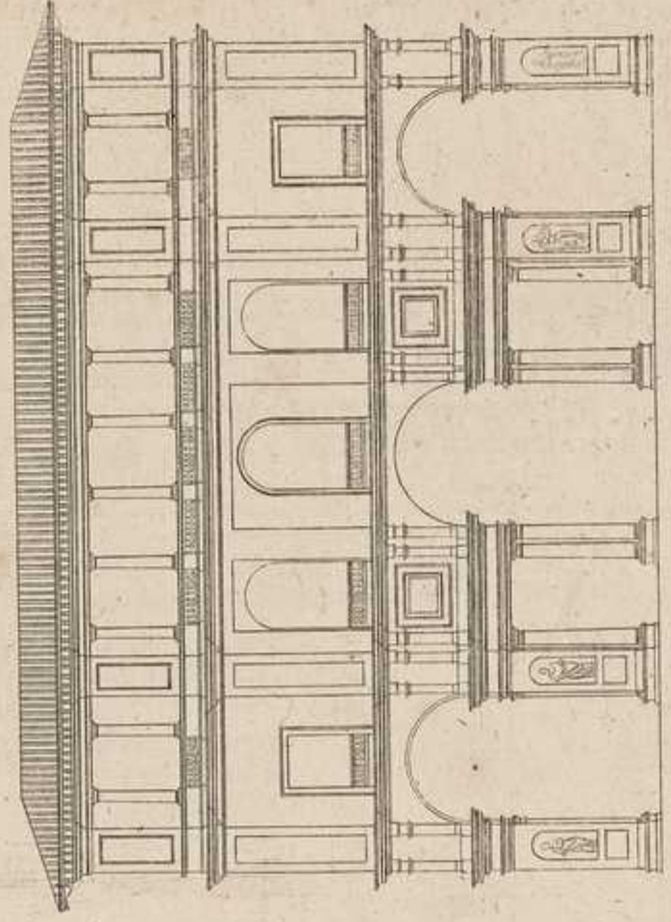
ELEVATION DU PALAIS DES OFFICES CÔTÉ DU FLEUVE.
