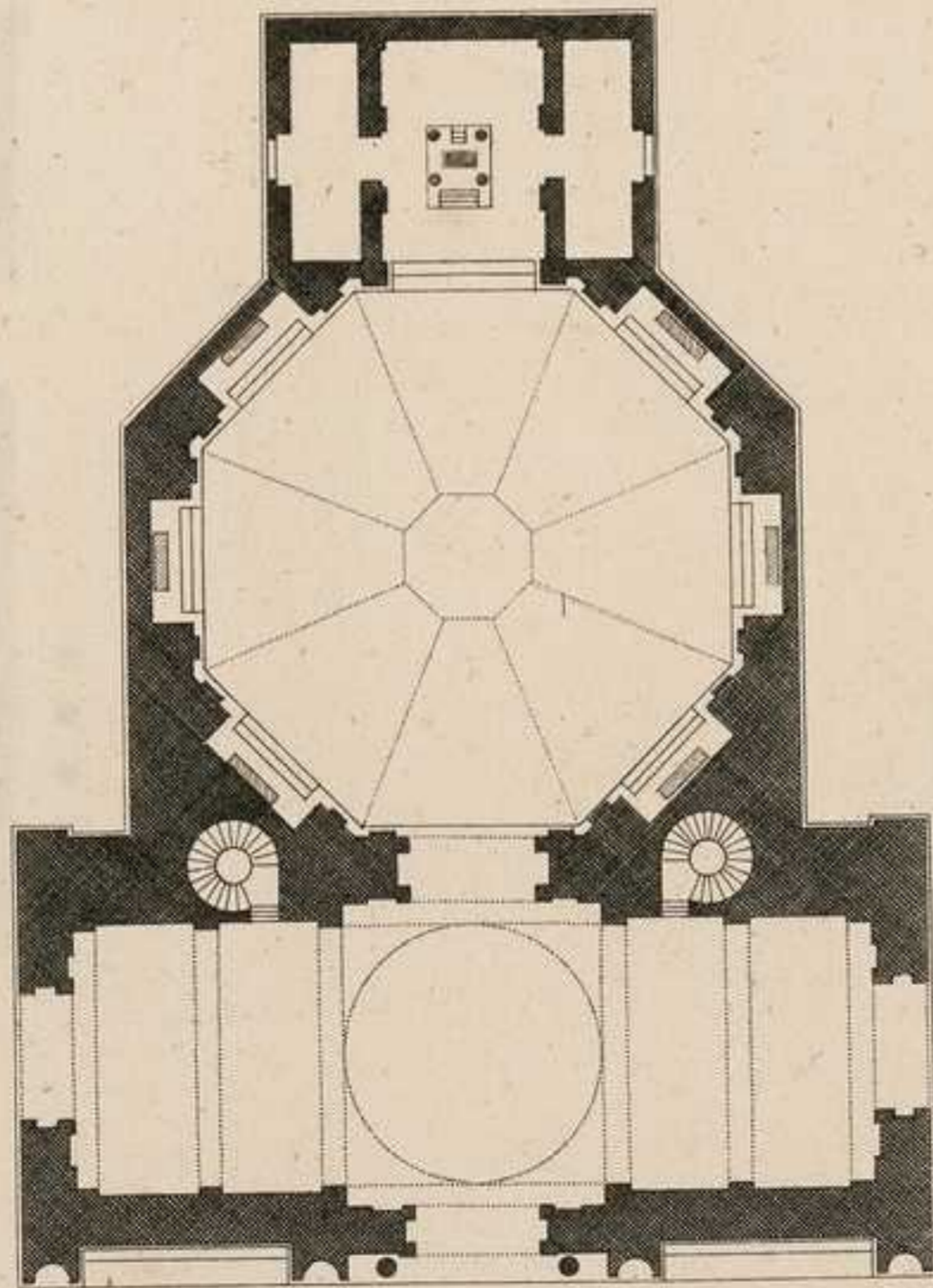
PLAN DE L'EGLISE DE L'UMILTA, A PISTOJA.
