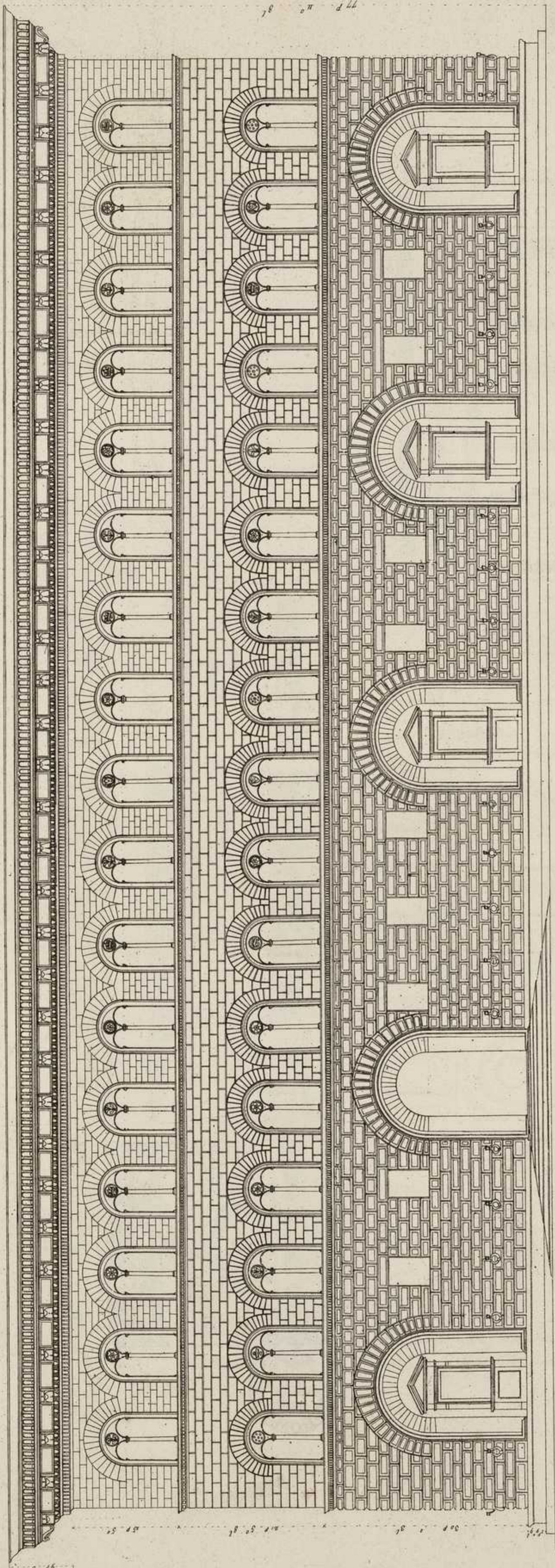
ÉLEVATION GÉOMÉTRALE DU PALAIS RICCARDI. DANS LA VIA LARGA, A FLORENCE.
