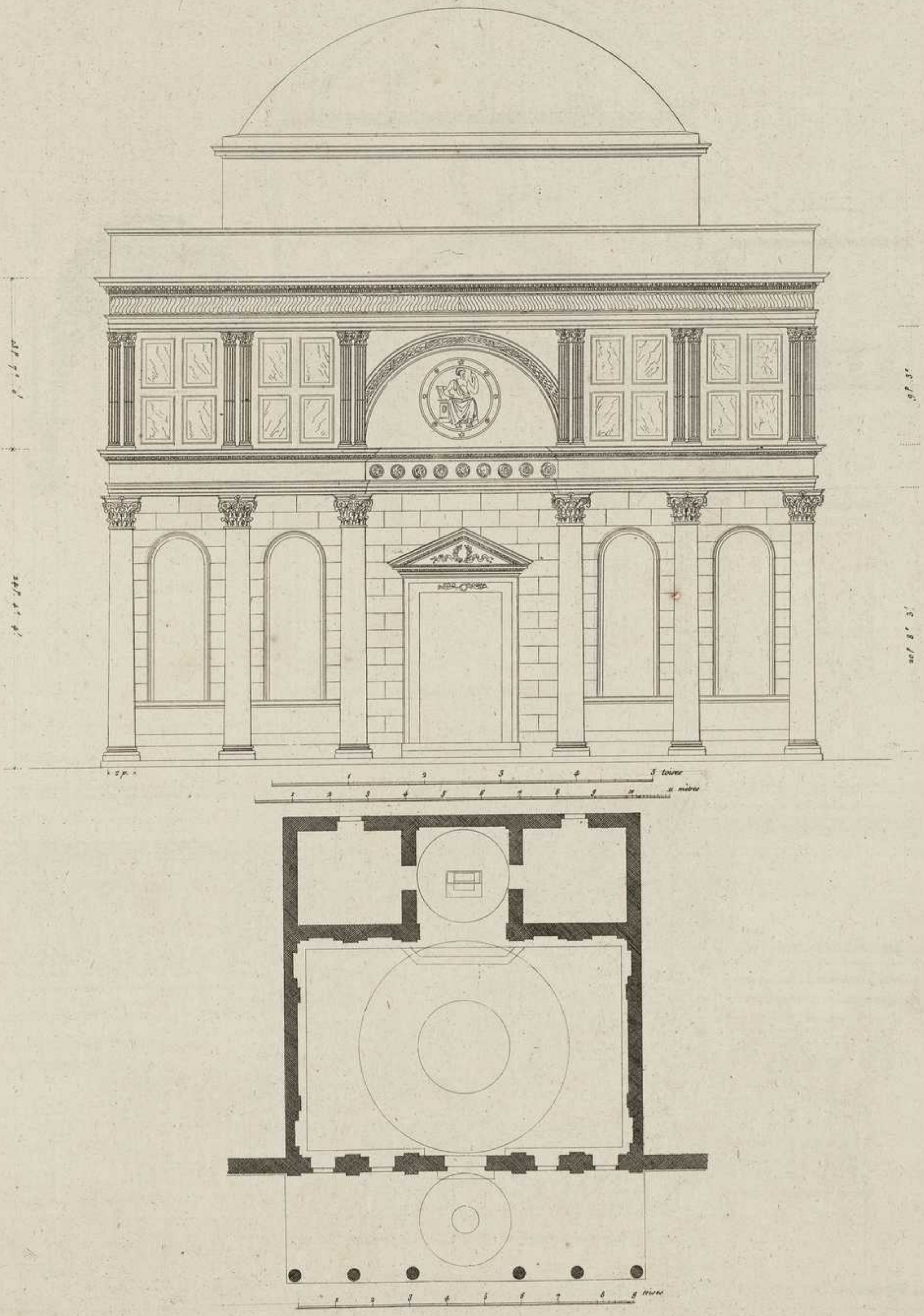
PLAN ET ELEVATION GÉOMÉTRALE DE LA CHAPELLE DES PAZZI DANS LE CLOÎTRE DE S T E CROIX, A FLORENCE.
