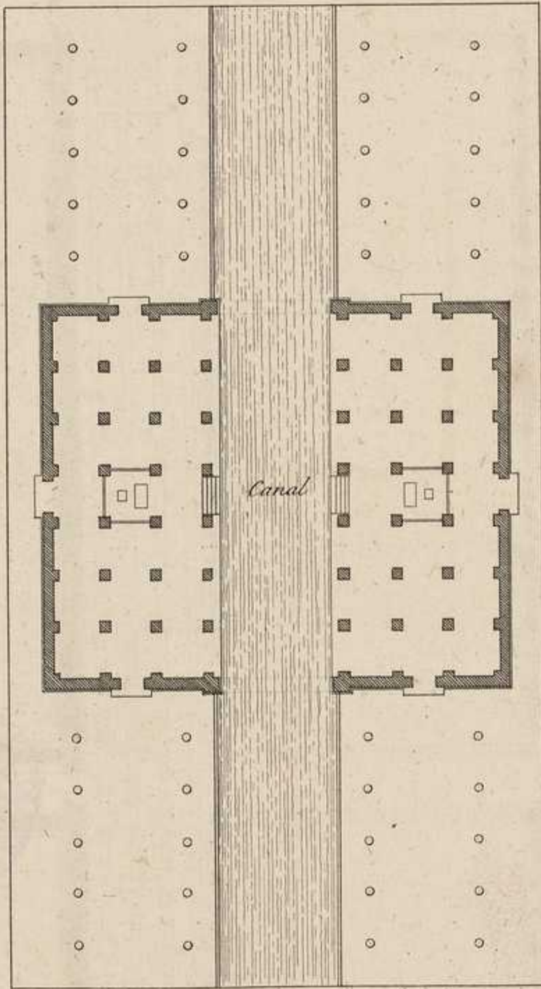
PLAN DE LA DOUANE PRÈS DE PISE.
