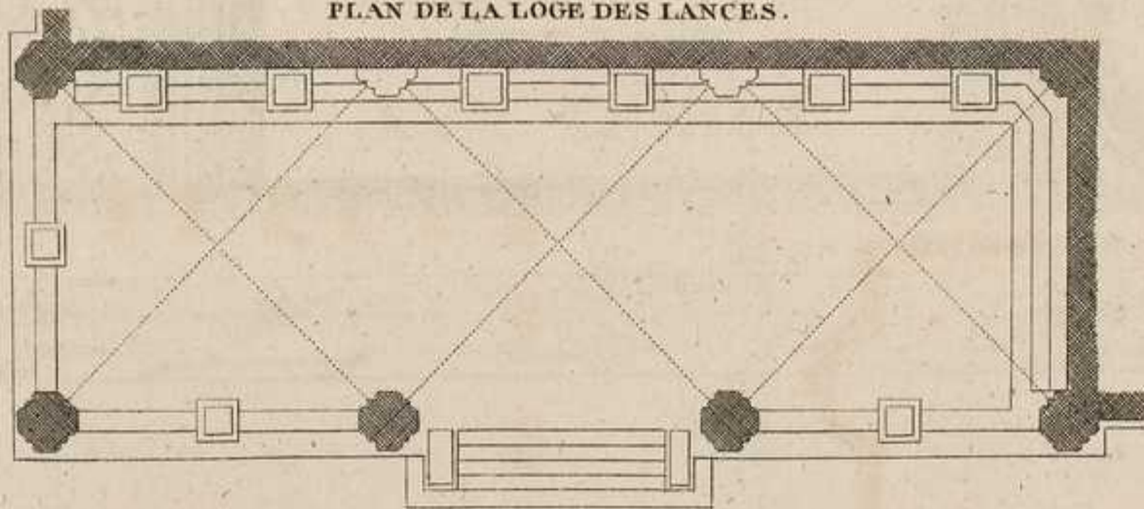
PLAN DE LA LOGE DES LANCES .
