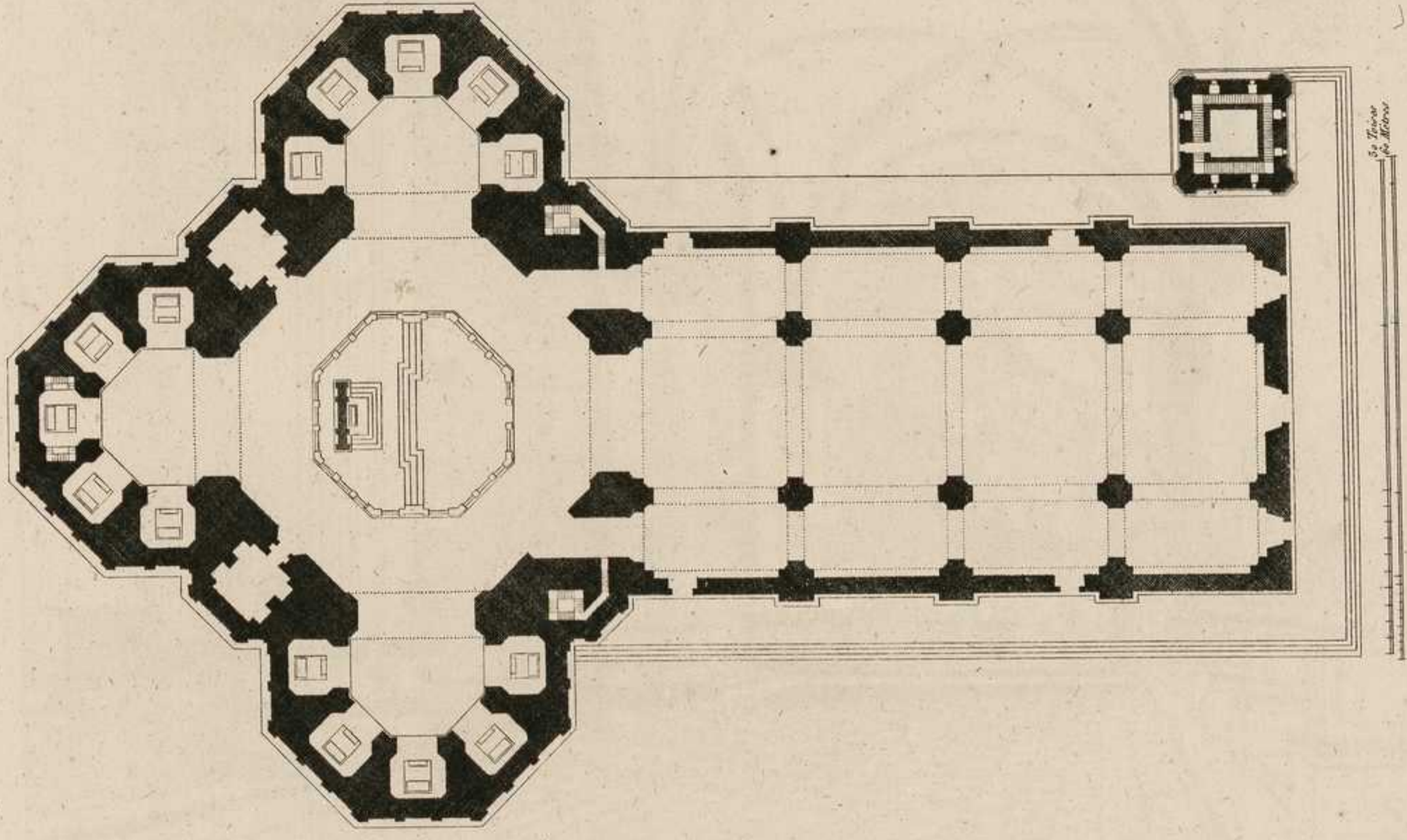
S T MARIE DES FLEURS A FLORENCE.
