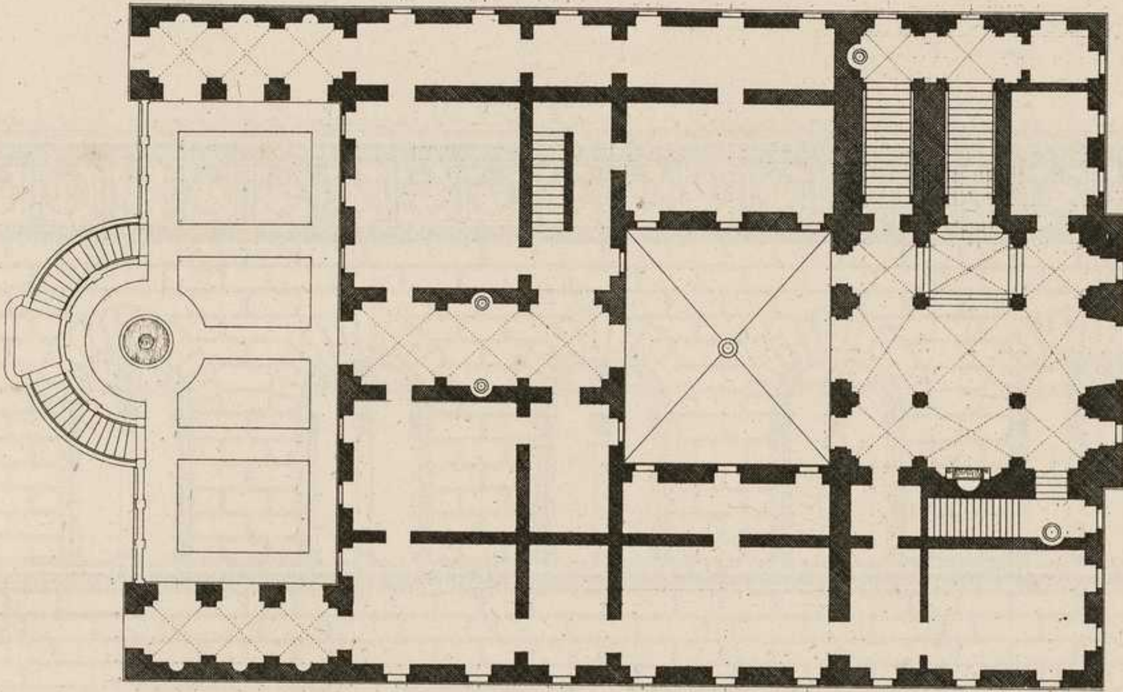
PALAIS SERGARDI A SIENNE
