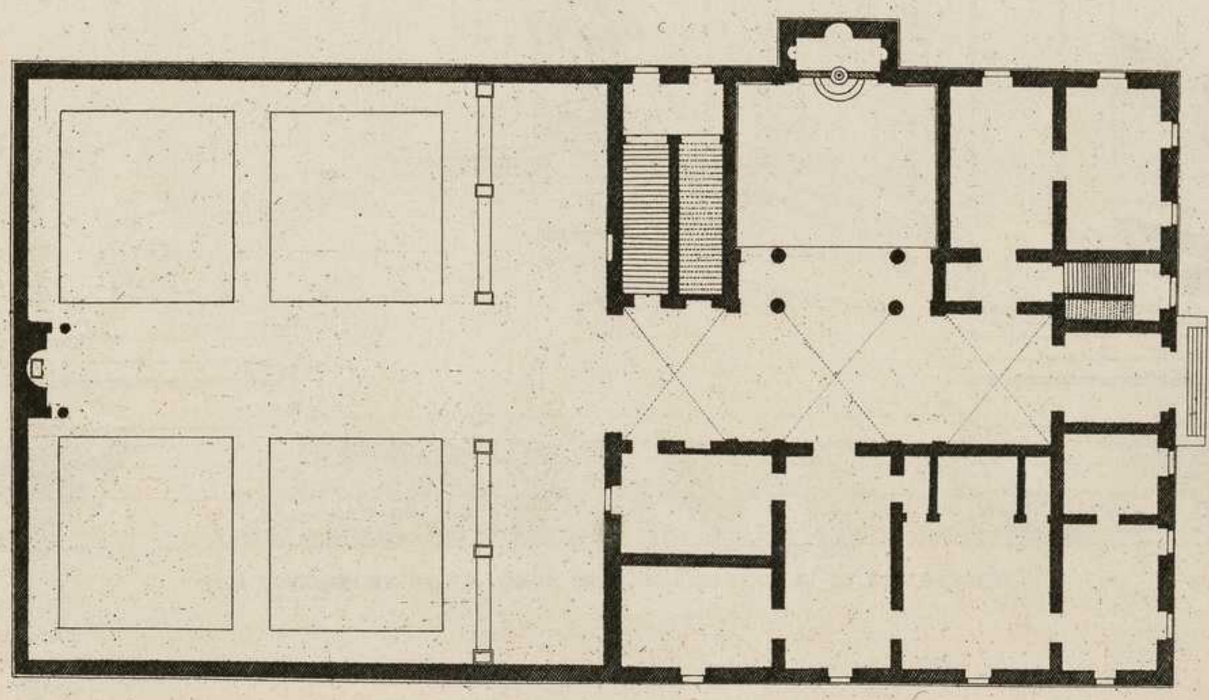
PALAIS PUCCI VIA DEI CRESCI A FLORENCE.
