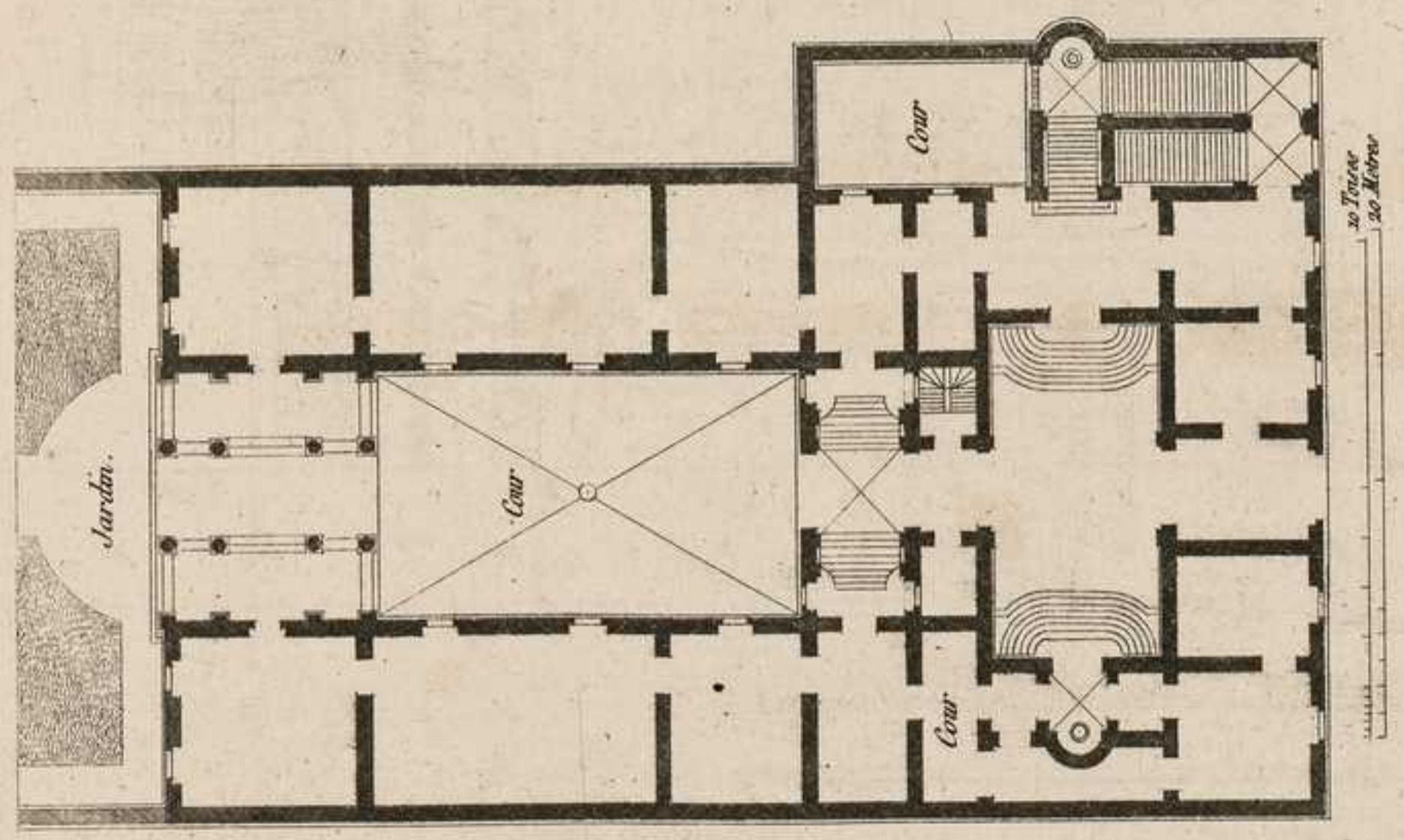
PLAN DU PALAIS CIMENES A FLORENCE.
