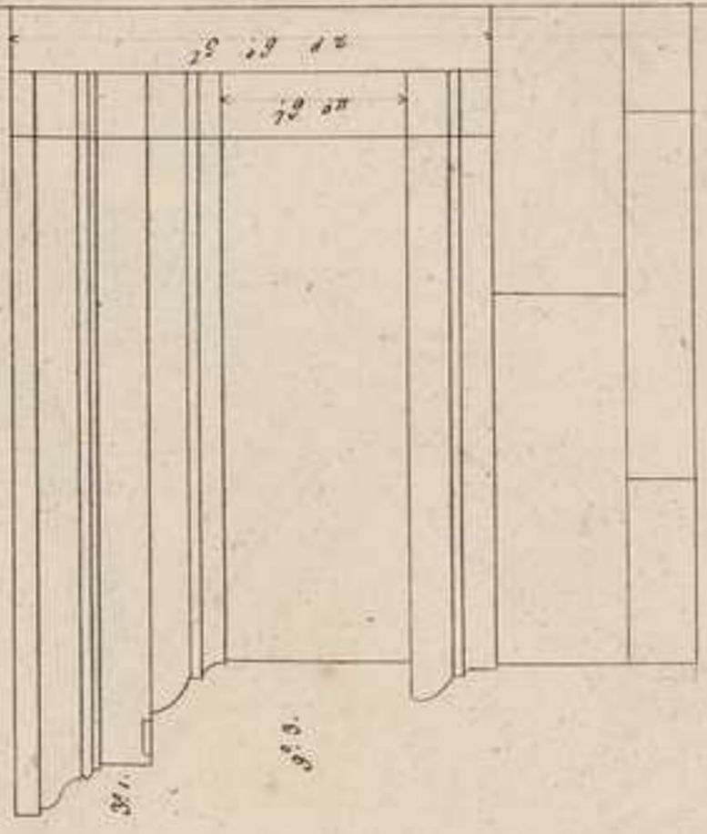
CORNICHE DU COURONNEMENT
