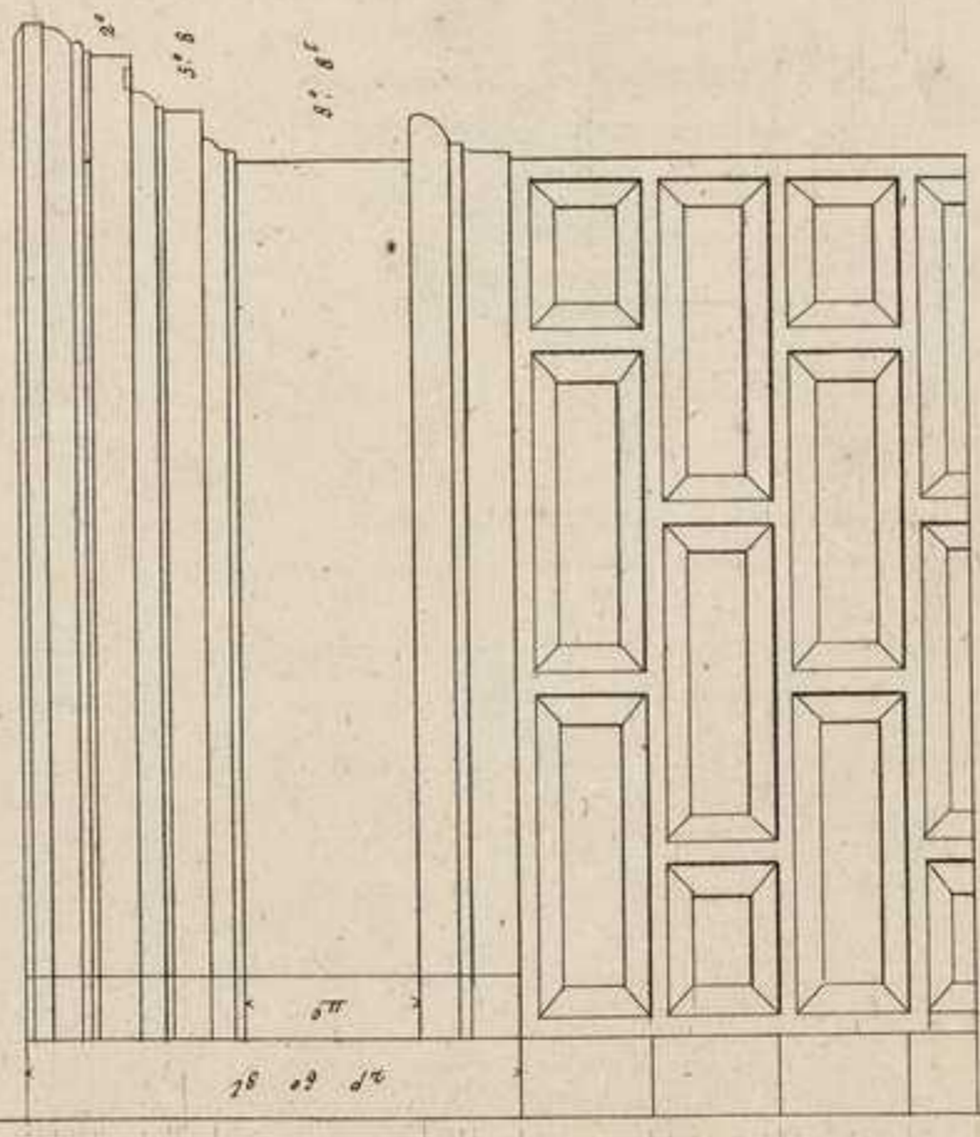
CORNICHE DU SOUBASSEMENT.
