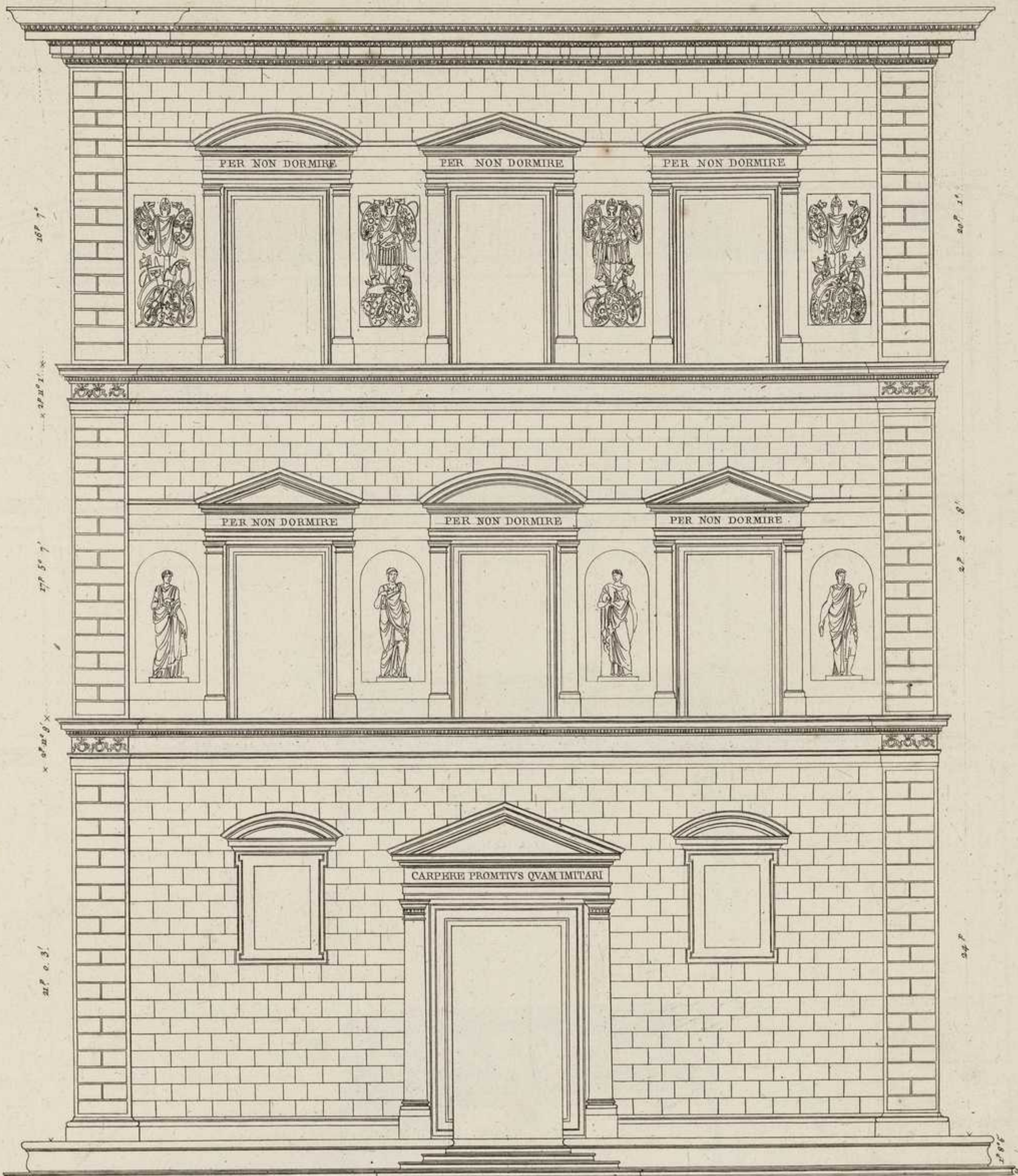
Echelle de l'Elevation 4 Toises 6 Mètres
