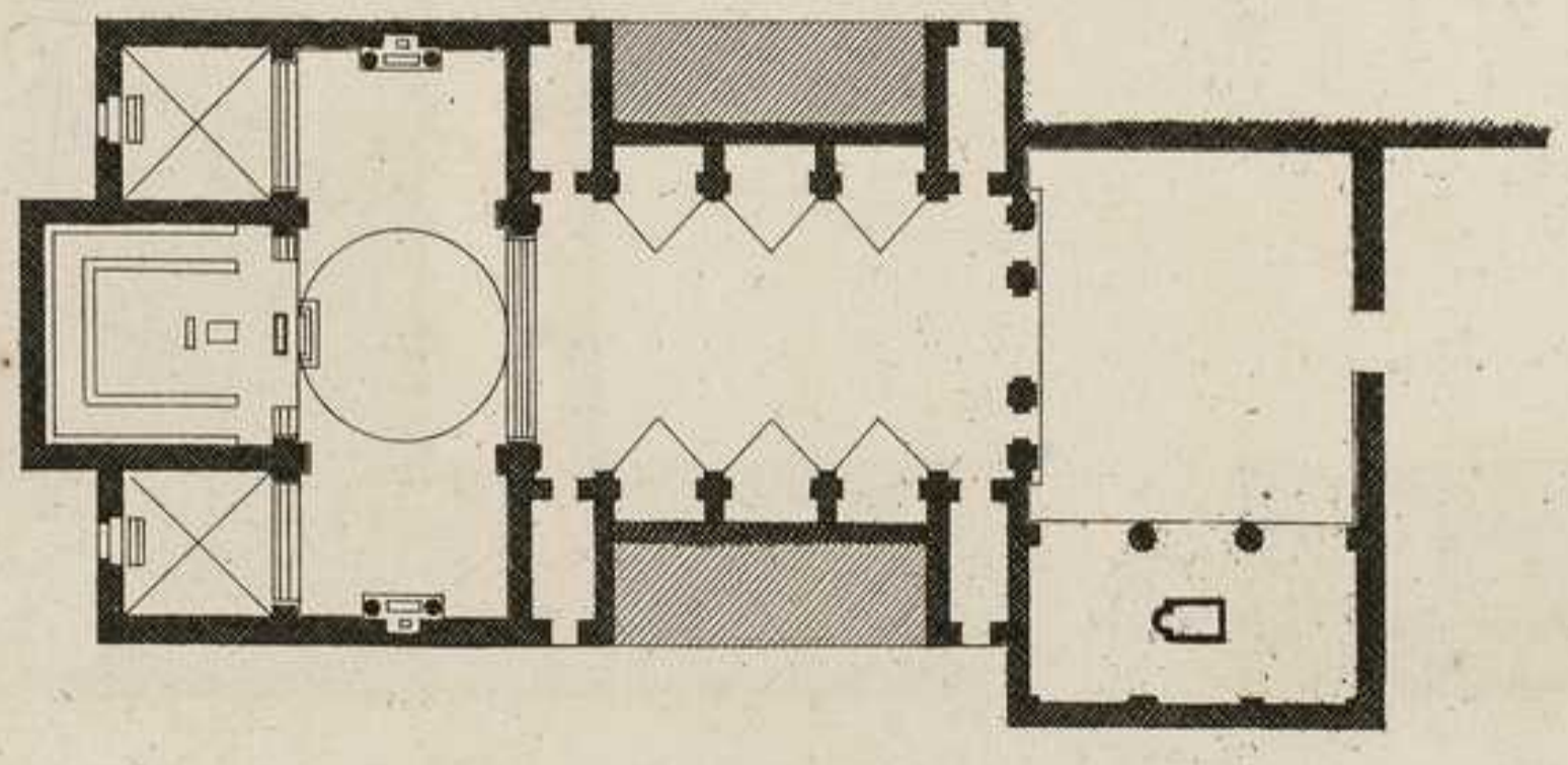
PLAN DE L'EGLISE DE S T FANCRASE, A FLORENCE
