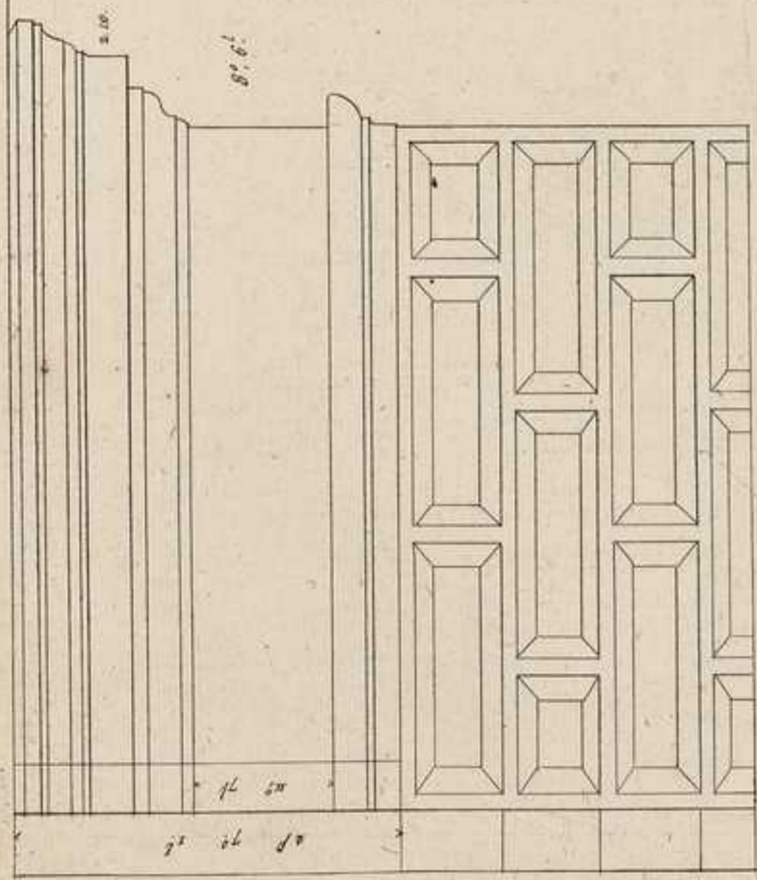
DÉTAILS DU PREMIER ÉTAGE.
