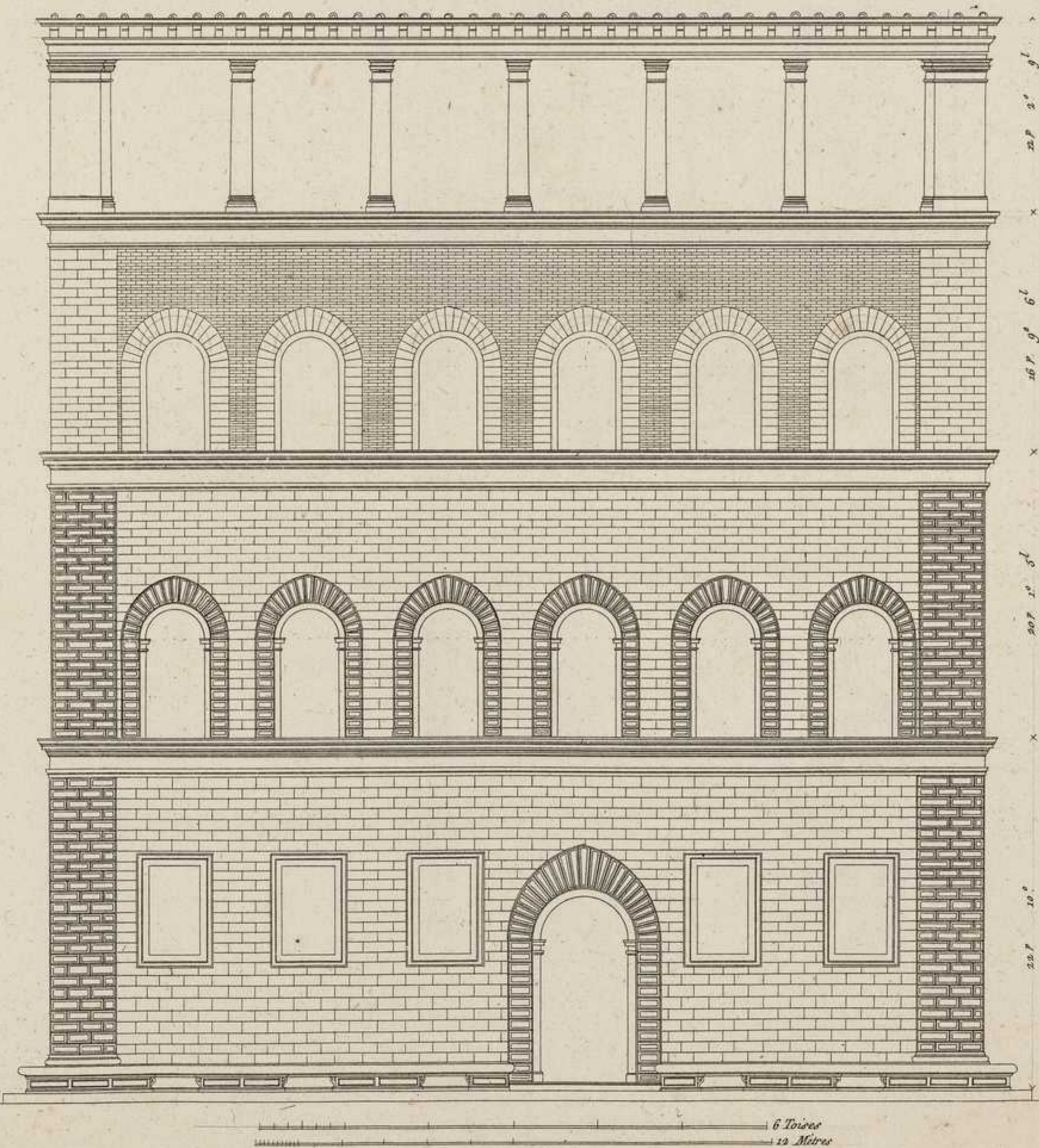
ELEVATION GEOMETRALE DU PALAIS NICOLINI, A FLORENCE
