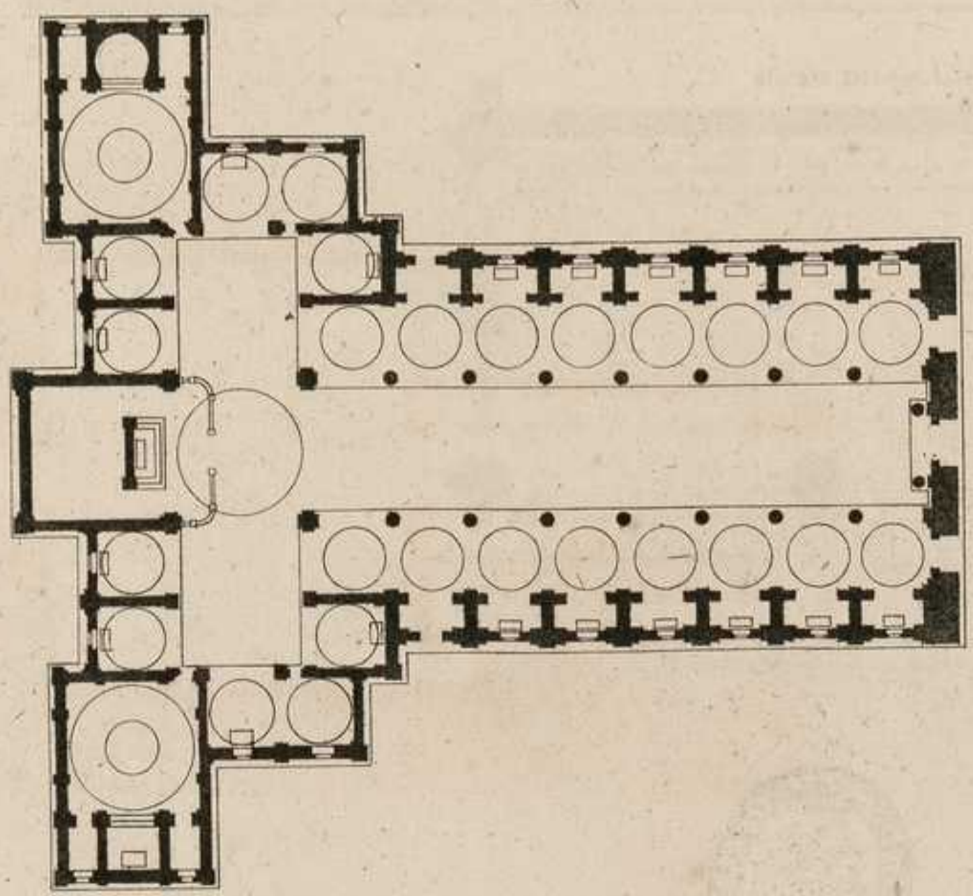
S T MARIE NOUVELLE A FLORENCE.
