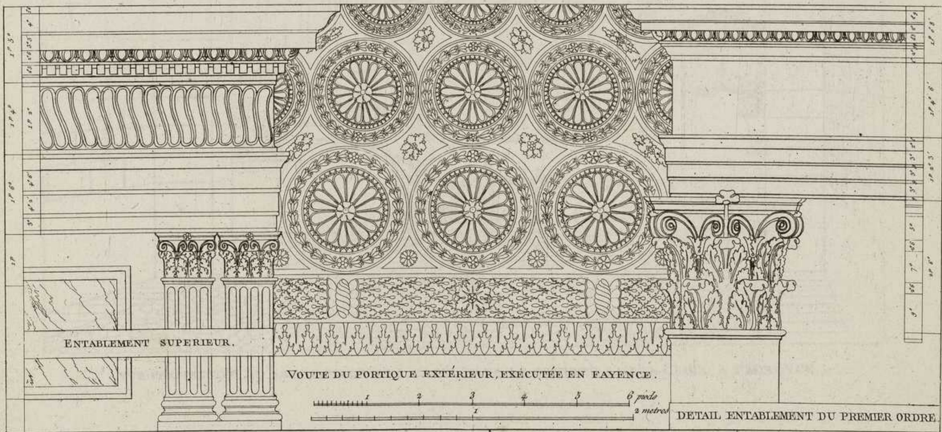
DÉTAILS DU PORTIQUE EXTÉRIEUR DE LA CHAPELLE DES PAZZI A FLORENCE.
