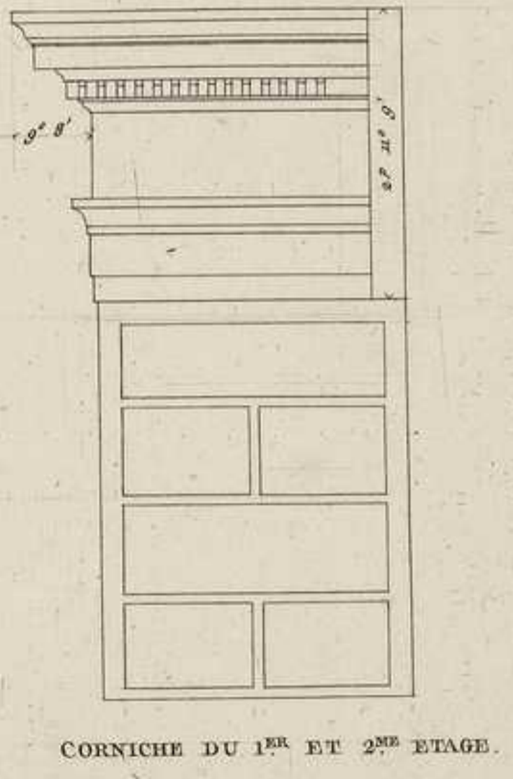
Echelle des détails 2 Mètres
