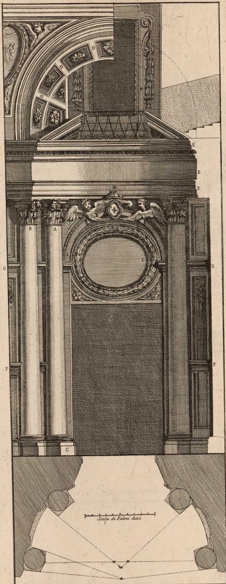
PROSPETTO INTERIORE DELLA PORTA PRINCIPALE DELLA CHIESA DI S. CARLO ALLE QUATTRO FONTANE
