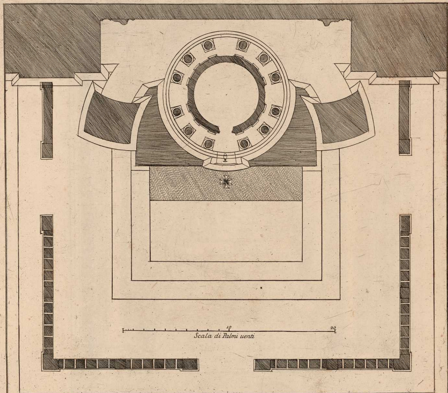
PIANTA DEL PRECEDENTE ALTARE E CIBORIO DELLA BASILICA VATICANA
