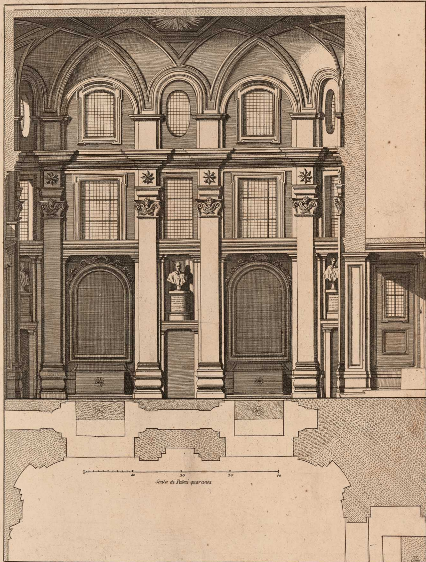
SPACCATO DELLA CHIESA DENTRO AL COLLEGIO DI PROPAGANDA FIDE ARCHITETTURA DEL CAVALIER BORROMINI
