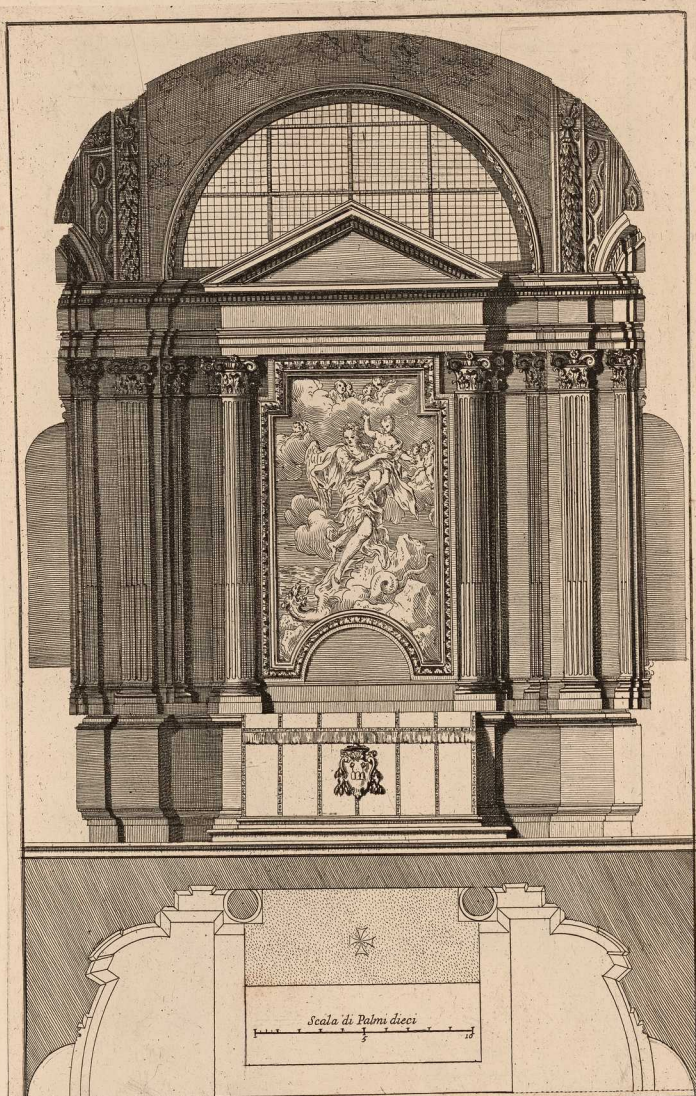
CAPPELLA DEL CARDINAL EAVSTO POLI ERETTA NELLA CHIESA DI S. GRISOGONO IN TRASTEVERE ARCHITETTURA DEL CAVALIER GIO. LORENZO BERNINI
