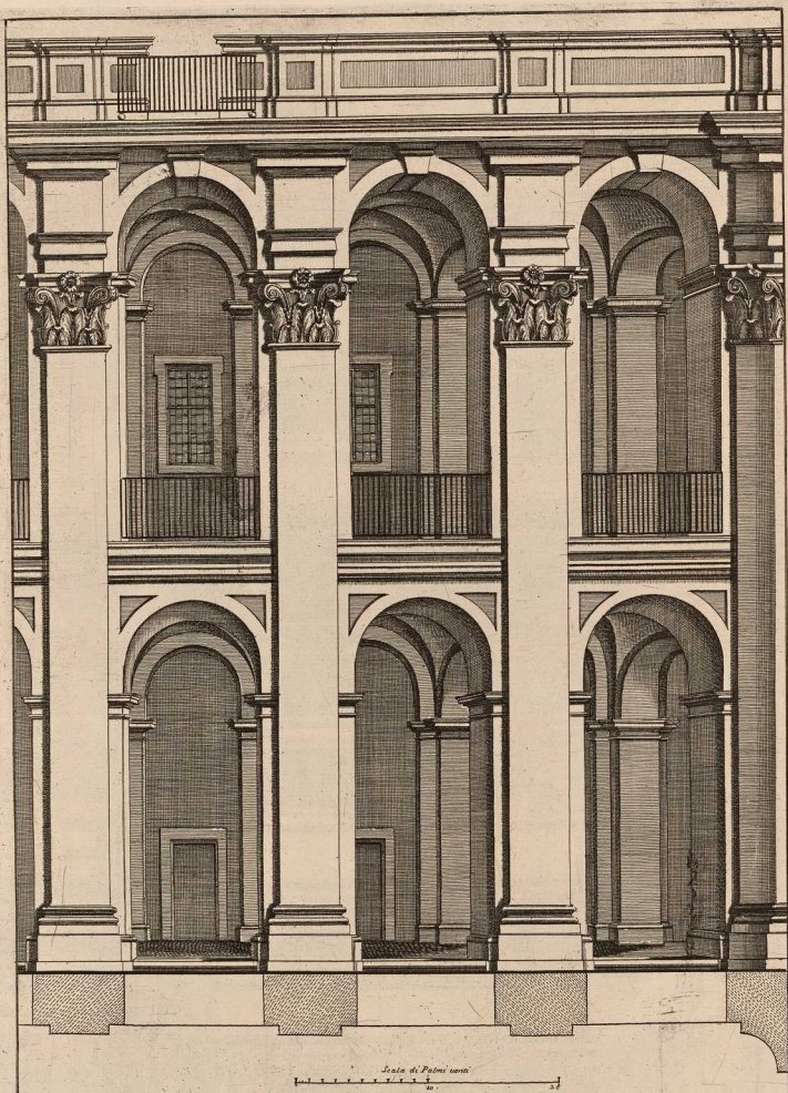
PARTE DEL CORTILE PRINCIPALE DELL' ABITAZIONE DE PADRI DI S. FILIPPO NERI IN S. MARIA IN VALLICELLA DETTA LA CHIESA N. VOVA ARCHITETTURA DEL CAVALIER BORROMINI
