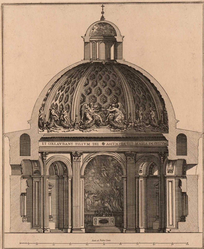
SPACCATO INTERIORE DELLA CHIESA DEDICATA ALLA S. MA VERGINE DELL'ARICCLA ARCHITETTURA DEL CAVALIER BERNINI
