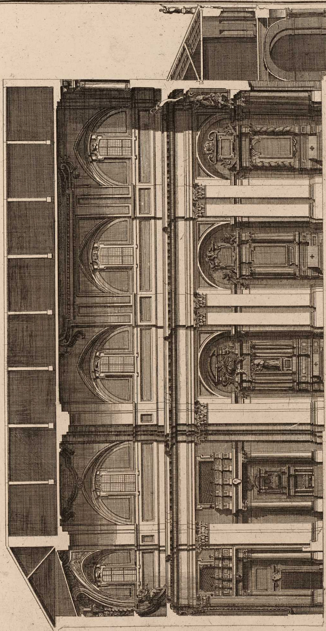
SPACCATO DELLA CHIESA DE SS. APOSTOLI DE PP. CONVENTUALI Architettura del Cavaliere Francesco Fontana.
