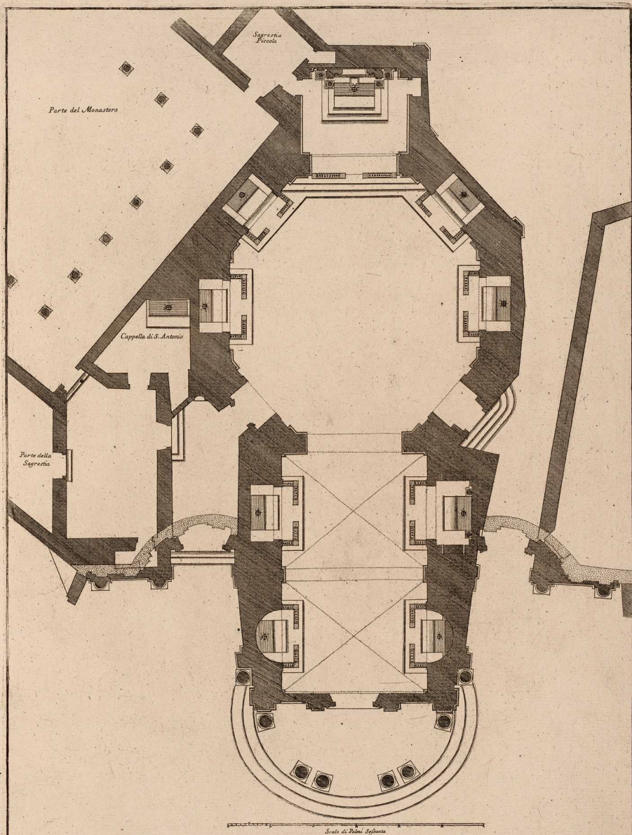
PIANTA DELLA CHIESA DI SANTA MARIA DELLA PACE DE CANONICI REGOLARI LATERANENSIS
