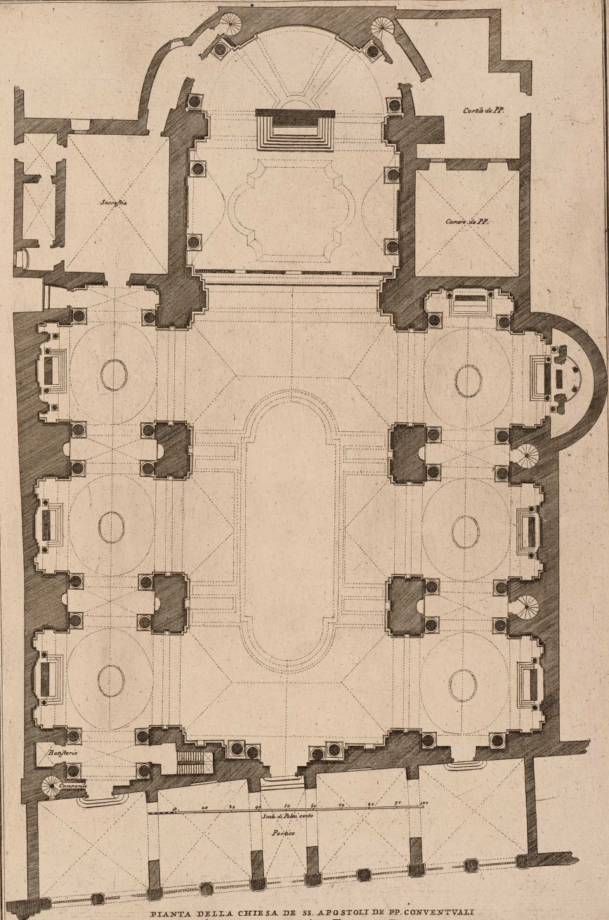
PIANTA DELLA CHIESA DE SS. APOSTOLI DE PP. CONVENTUALI Architettura del Cavaliere Francesco Fontana
