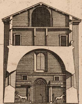
Prospetto interiore di detto Stallone
