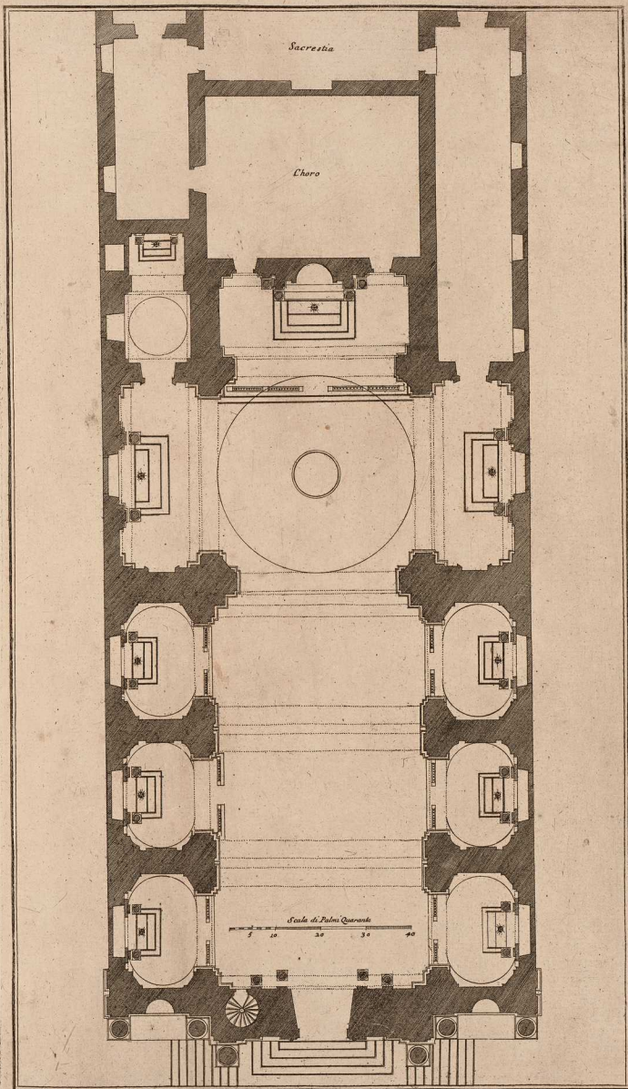
PIANTA DELLA CHIESA DI S. NICOLA DA TOLENTINO A CAPO LE CASE Nella Stamperia di Domenico De Ricci. Disegno di Gio: Giacomo In. Roma alla Pace con Privilegio del Sommo Pontefice. S
