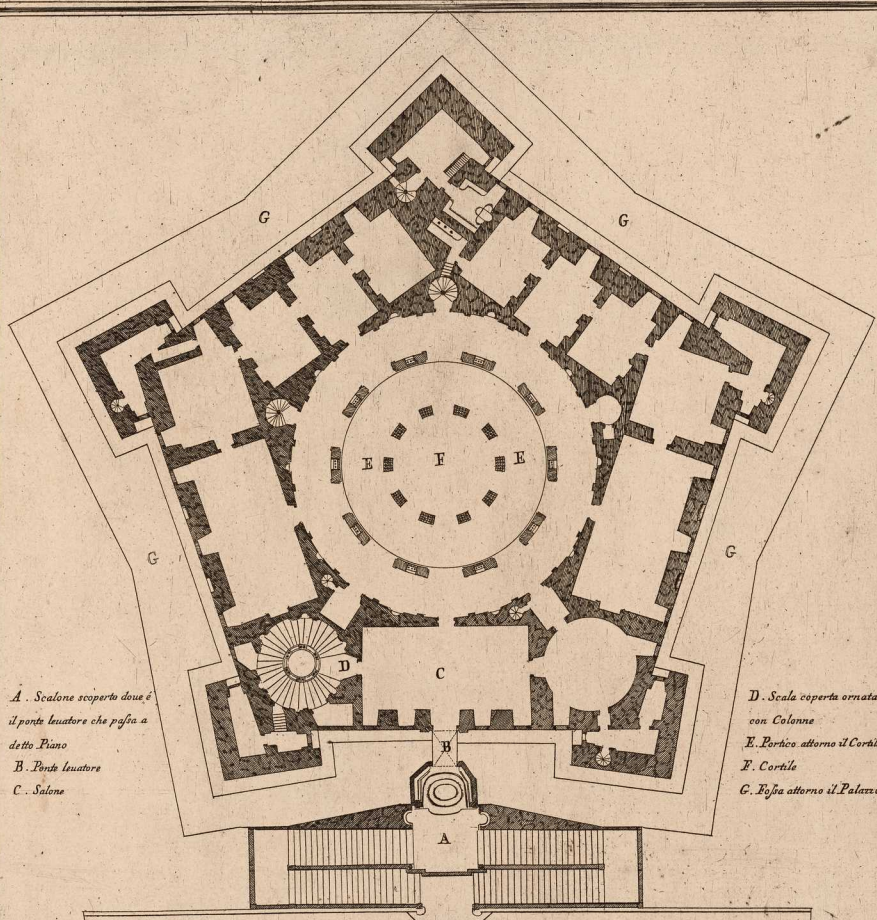
PIANTA DEL PIAN TERRENO DEL PALAZZO DI CAPRAROLA
