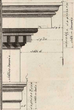
Architrave fregio e Cornice A.
