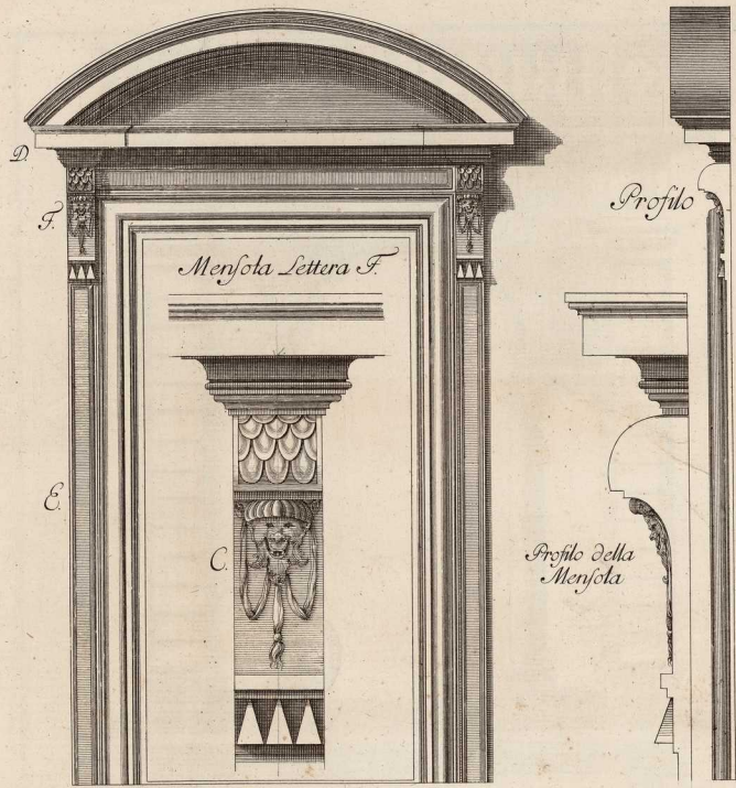
Modine delli Stipiti lettera E.
