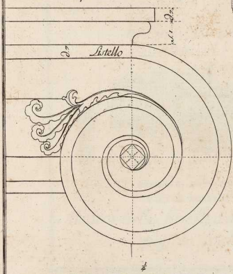
Scala di mezzo braccio per la Voluta
