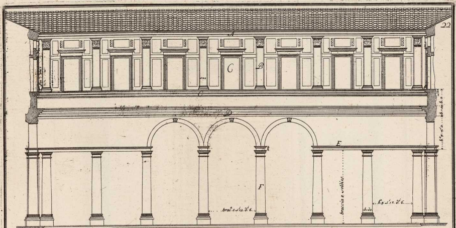
Aspetto del primo, e secondo Ordine che corrisponde alla sottoporta Pianta segnata A. B
