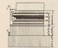
Dimostrazione delli Modini del passato foglio N. 3 di dentro la Libreria Laurenziana.
