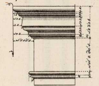
Capitello di Alatri A.
