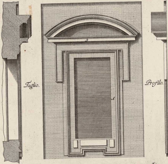
Modine delli Stipiti lettera A.
