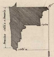
Scala di braccia due per li present i Modini.
